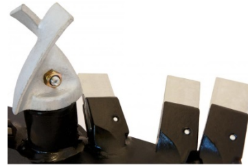
Boorvijzels, steeds met vervangbare slijtpunten!
